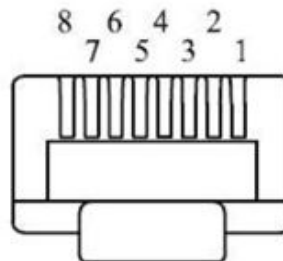
T568A
