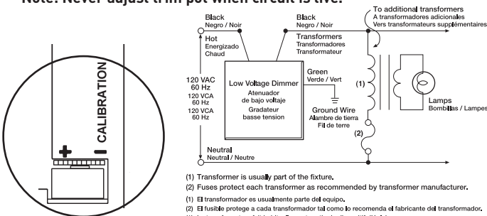
Wiring Diagram Diagrama de Cableado / Schéma de câblage
