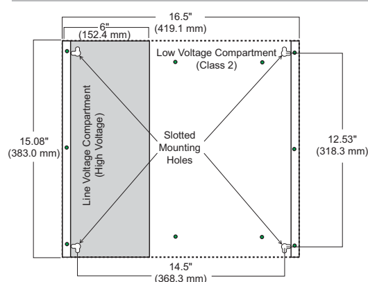
LP8 Dimensions
