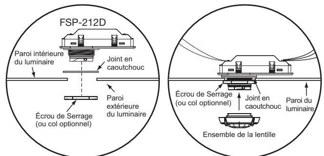
Montage à collet fileté
