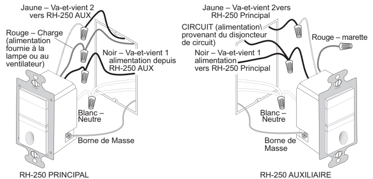
Fig. 4 : Étape 4a. Orientation du détecteur, branchement des fils et montage de boîtier mural
