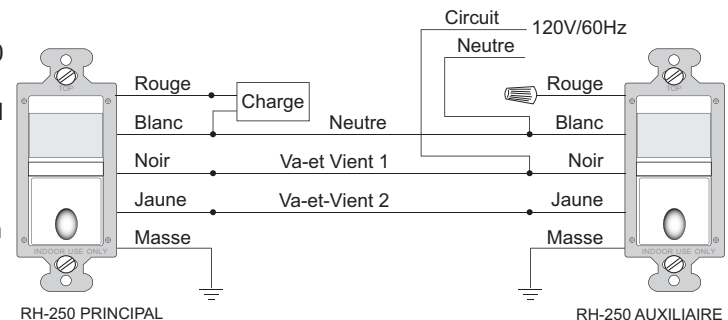
Fig. 5 Étape 4a. Schéma de câblage de référence
