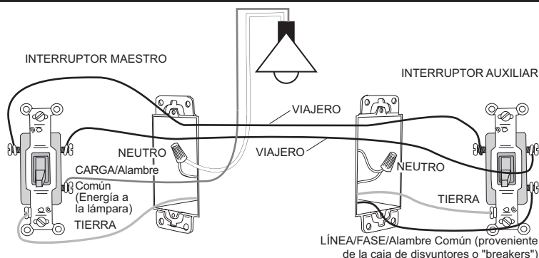
Fig. 2: Conexión típica de dos interruptores de 3 vías
