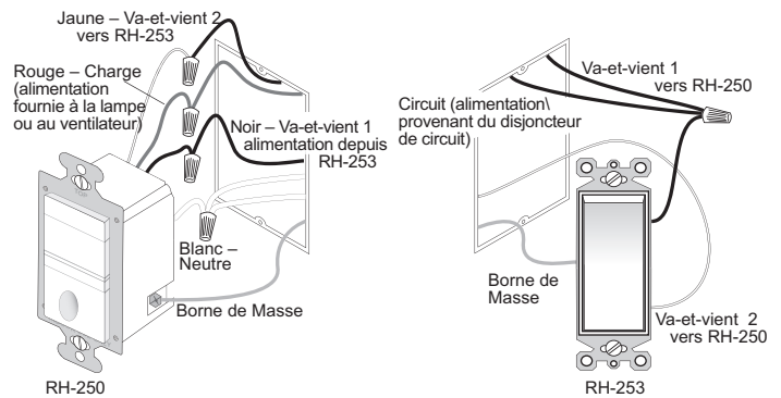
Fig. 6 : Étape 4b. Orientation du détecteur et branchement des fils pour le fonctionnement à 3 voies avec un interrupteur mural instantané RH-253
