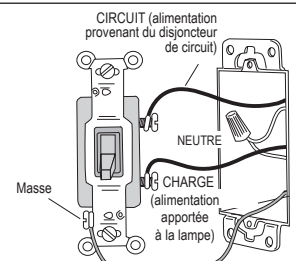
Fig. 2 : Câblage typique d'un commutateur unipolaire
