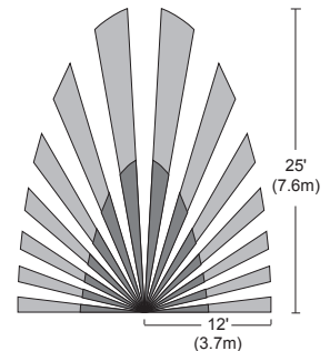
Fig. 1 : Zone de couverture du détecteur
