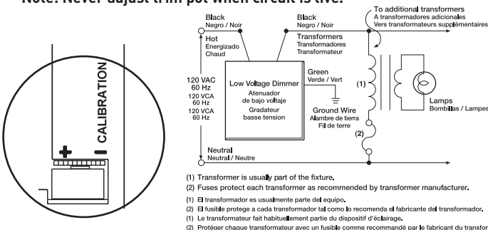
Wiring Diagram Diagrama de Cableado / Schéma de câblage
